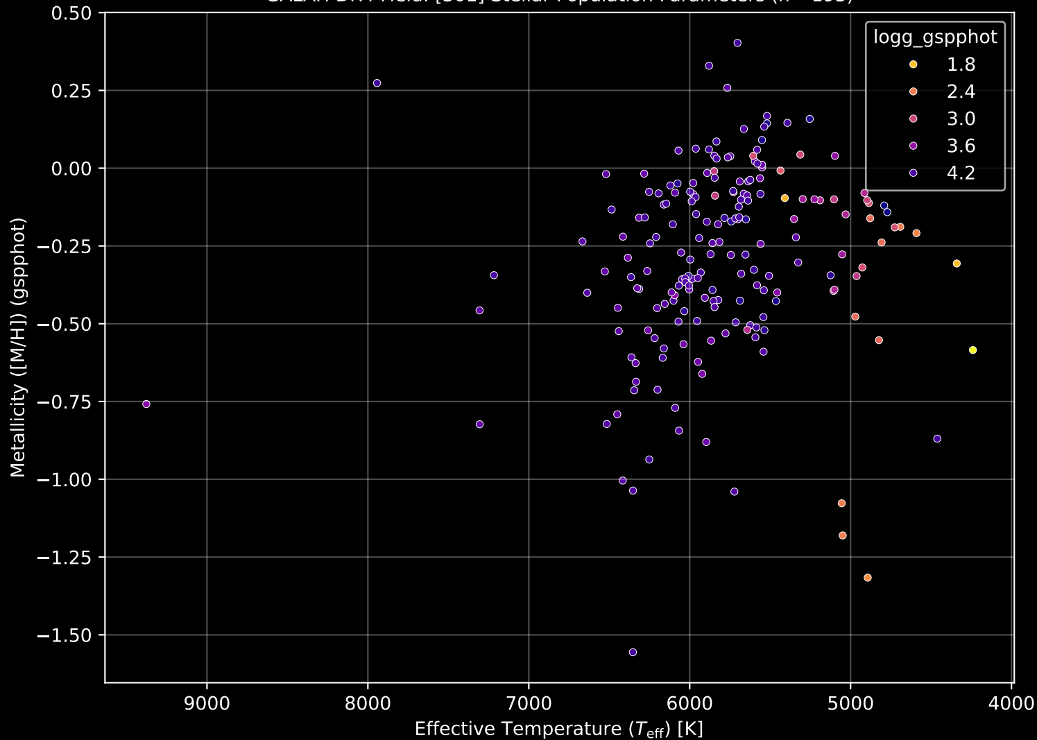
GALAH DR4 Field: [301] Stellar Population Parameters (n= 193)
